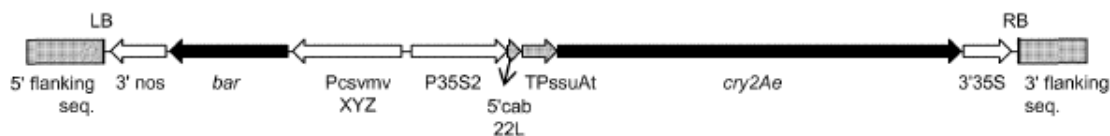
図5 GHB119に移入されたDNAの構成図
